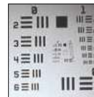
Κατασκευαστής B (20.16 LP/mm)
